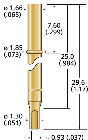
S 100.00-L Solder Cup
