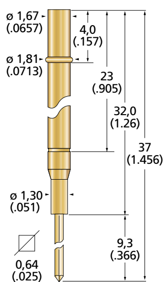
S 100.04-WI Wire-Wrap-Post
