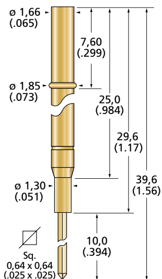
S 100.00-W Wire-Wrap-Post
